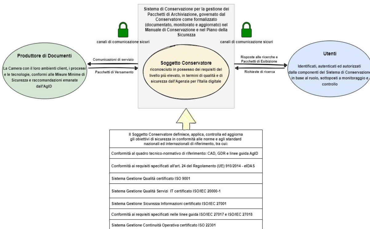
Applicazione sicura del modello di riferimento dello standard OAIS
